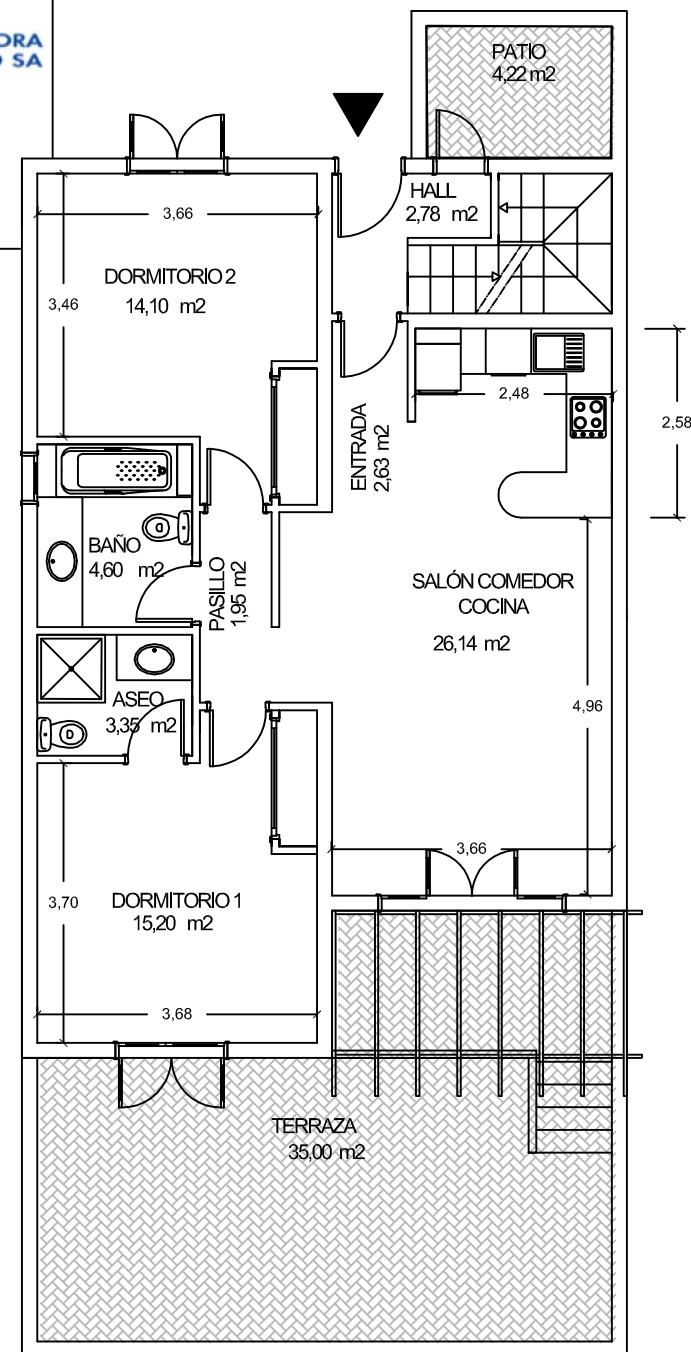
PLANTA BAJA
