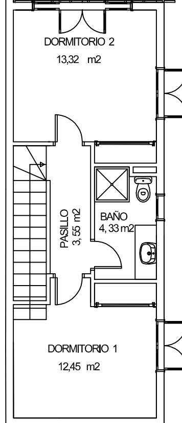
PLANTA BAJA
