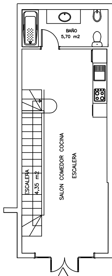
PLANTA SEMIBAJA
